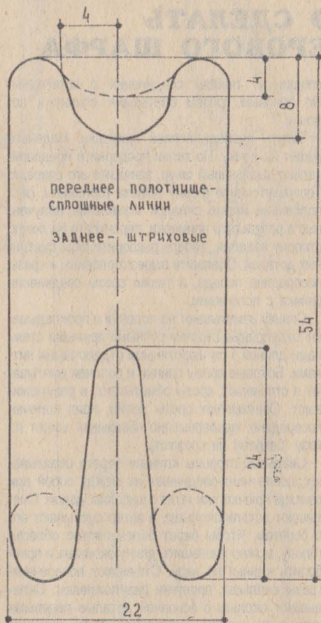
ВЫКРОЙКА ПОЛЗУНКОВ
